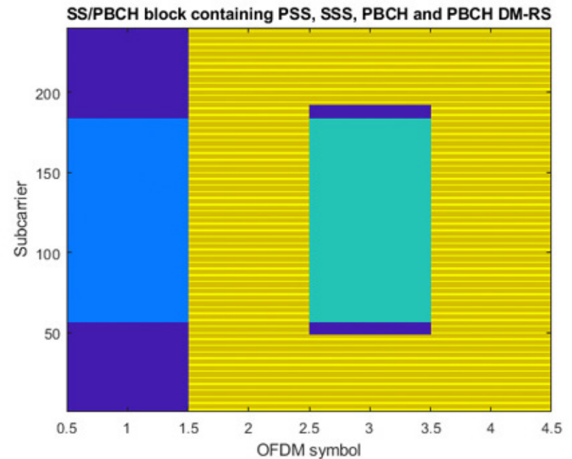
包括主要和辅助同步序列、广播信道和相关 DMRS 的 5G SSB 资源网格的详细视图。
