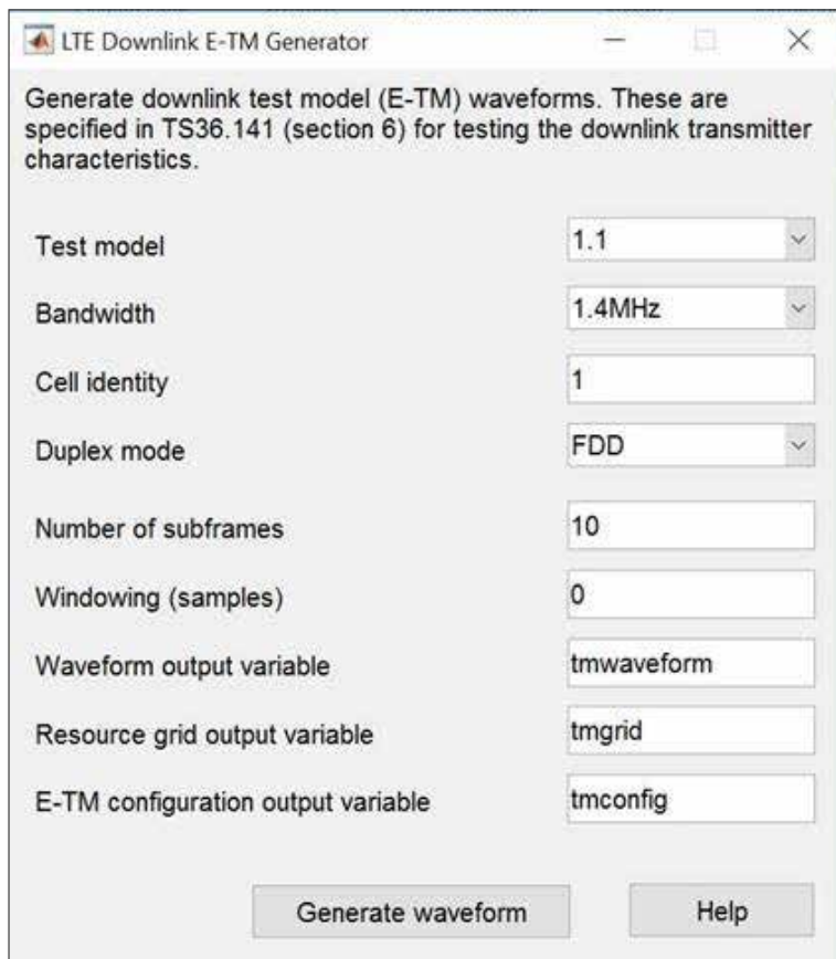
LTE 下行链路测试模型 (E-TM) 波形的生成 (左) 和分析 (右)
