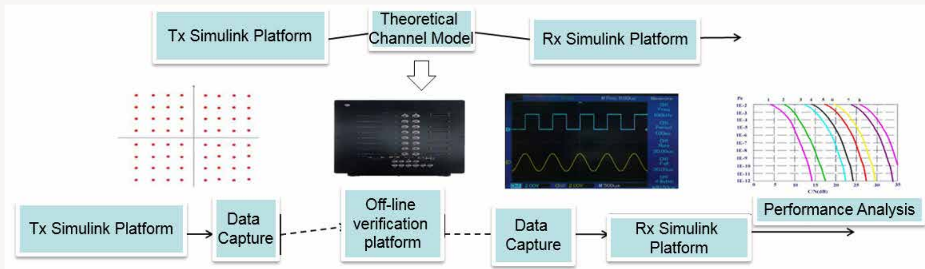
使用 Simulink 进行超高速算法仿真和离线验证
