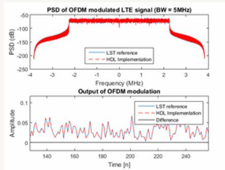
验证 OFDM 调制的 HDL 实现
