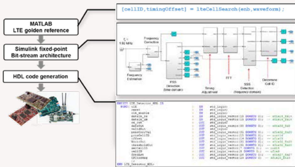
用于 LTE 小区搜索的 MATLAB 参考代码 (顶部)，以及用于设计和生成该算法的 HDL 实现的工作流程 (底部)
